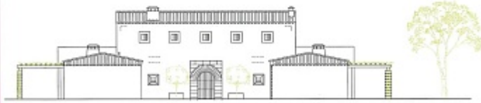
ALZADO POSTERIOR
